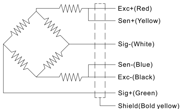
Wiring Code@Clockwise
