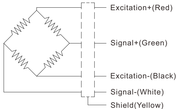
Wiring Code@Clockwise
