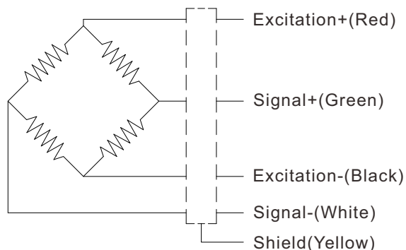
Wiring Code@Clockwise
