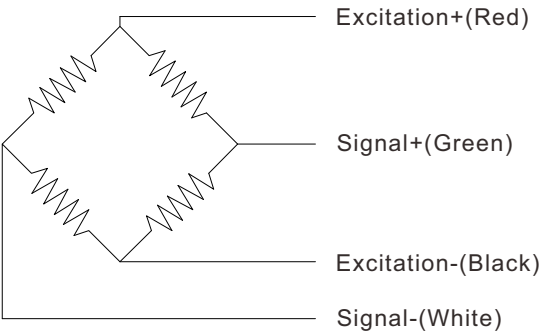
Wiring Code
