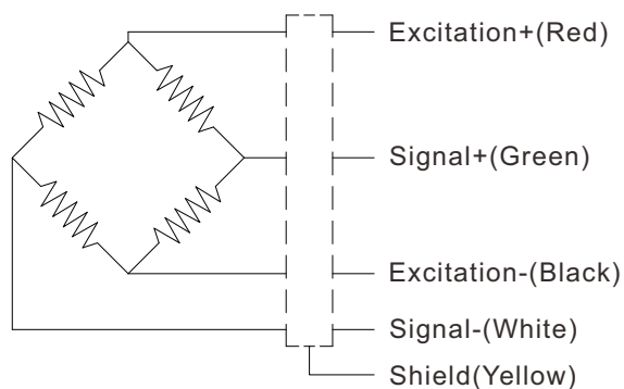
Wiring Code
